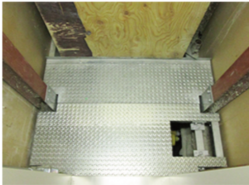
シャフト開口部塞ぎ金物
